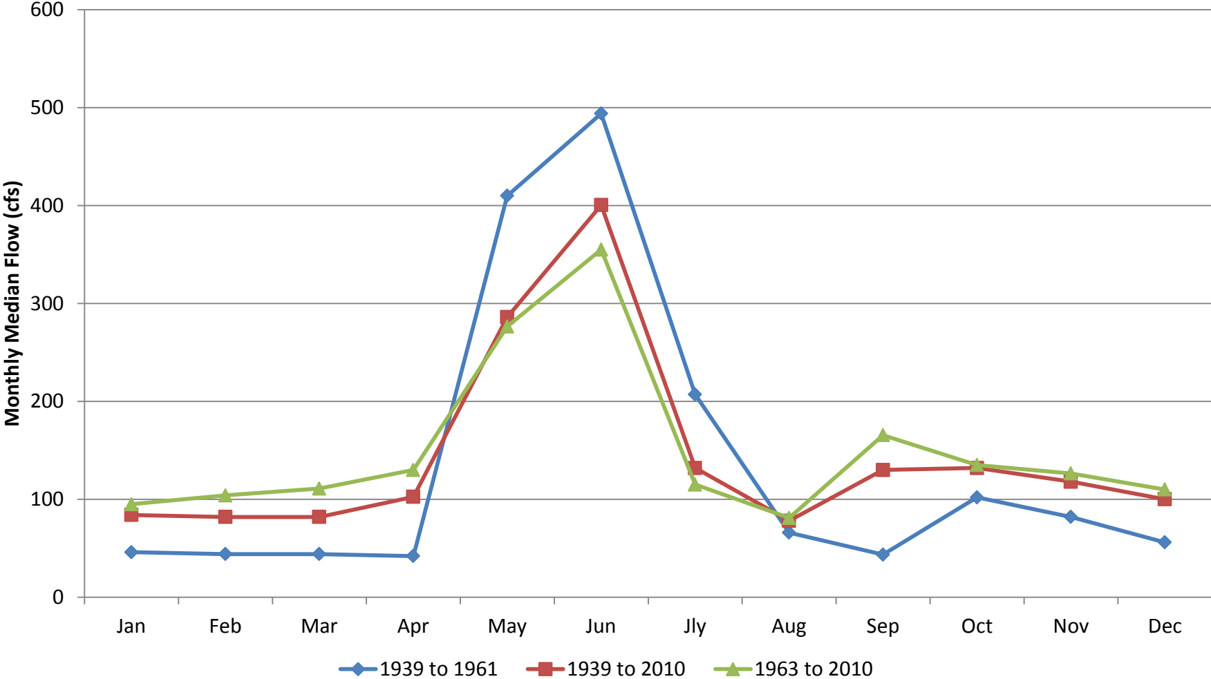
USGS 08088000 Brazos Rv nr South Bend, TX Monthly Medians
