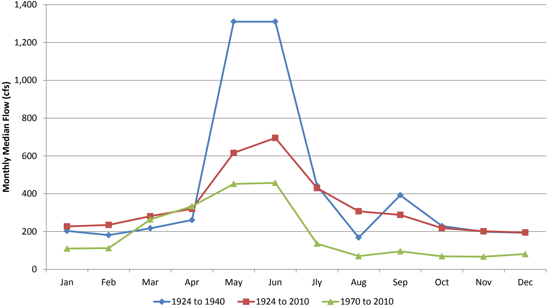
USGS 08091000 Brazos Rv nr Glen Rose, TX Monthly Medians
